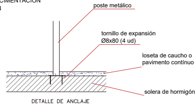
ESQUEMA DE CIMENTACIÓN EN HORMIGÓN
