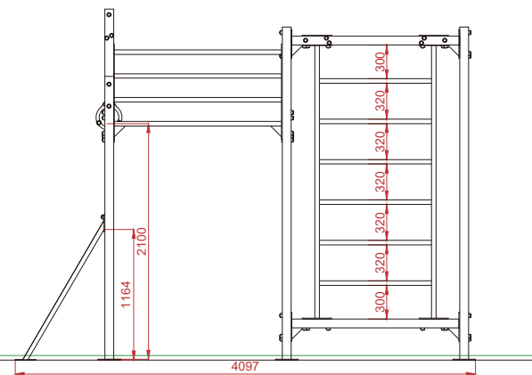
PERFIL
