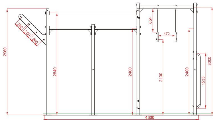
ALZADO
