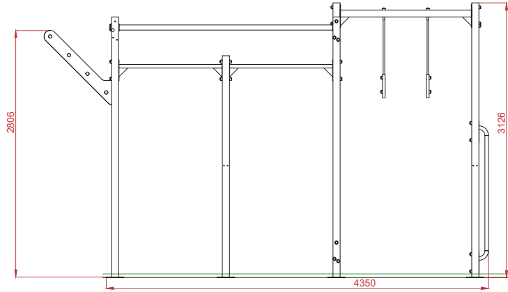
ALZADO
