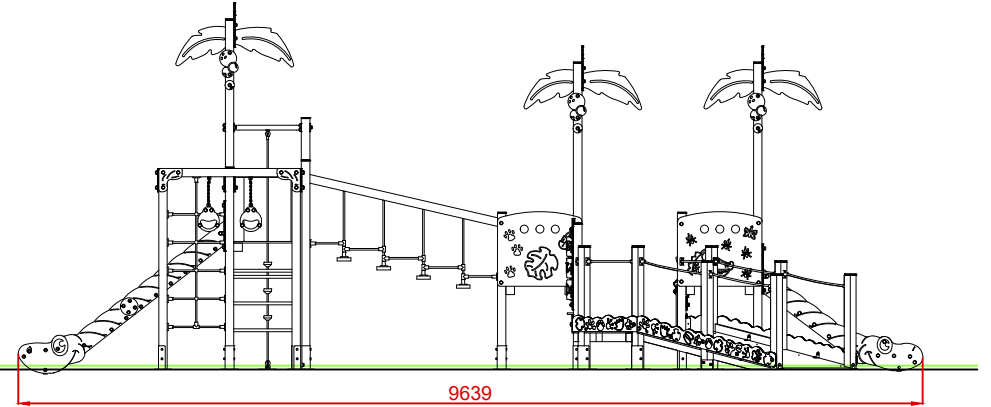
PERFIL IZQUIERDO
