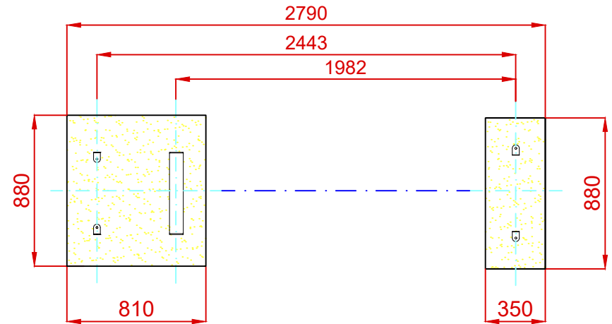
PLANTA CIMENTACIÓN
