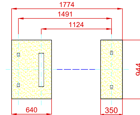
PLANTA CIMENTACIÓN
