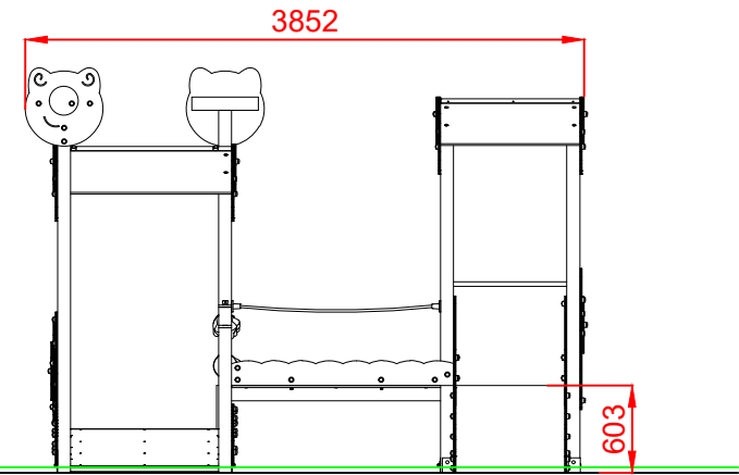
PERFIL IZQUIERDO
