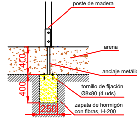
ESQUEMA DE CIMENTACIÓN EN ARENA
