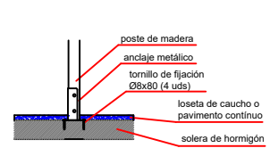
ESQUEMA DE CIMENTACIÓN EN HORMIGÓN
