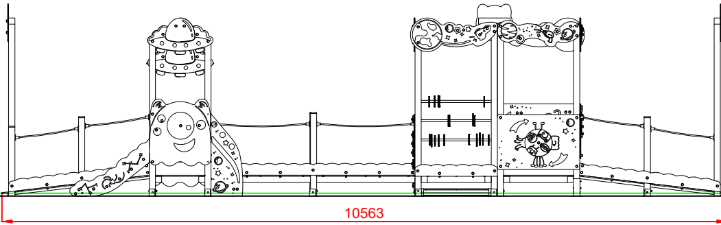
ALZADO
