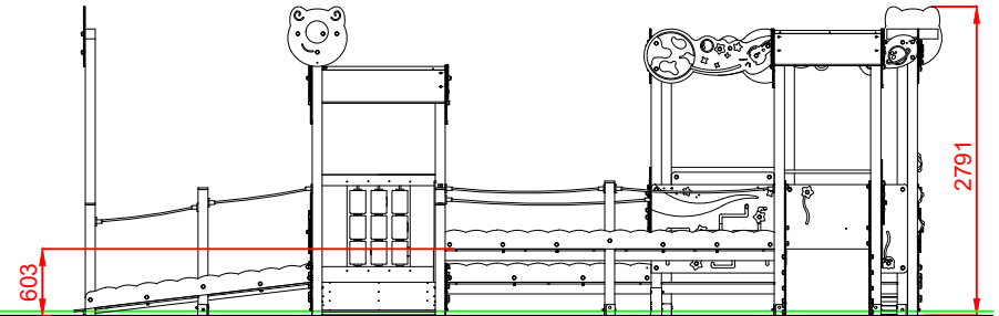
PERFIL IZQUIERDO
