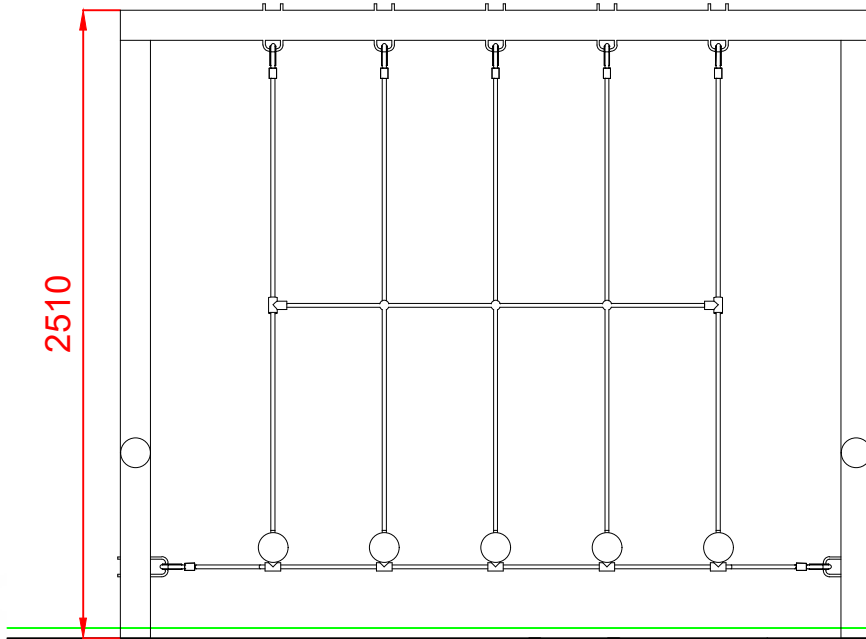
ALZADO
