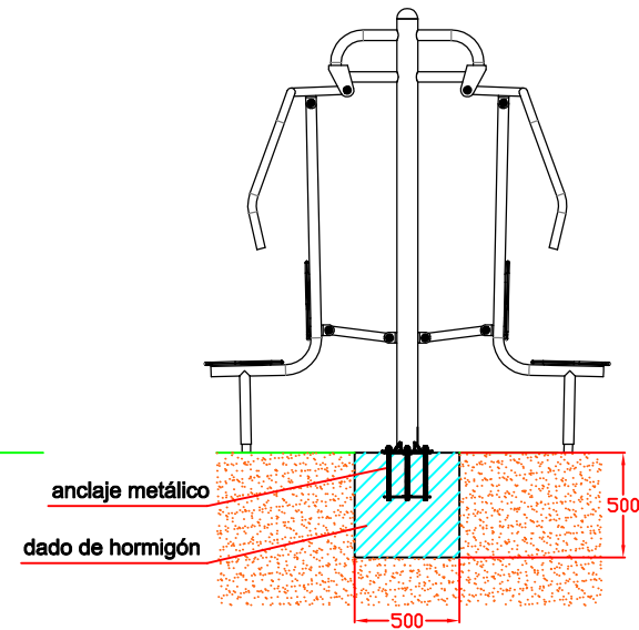
CIMENTACIÓN
