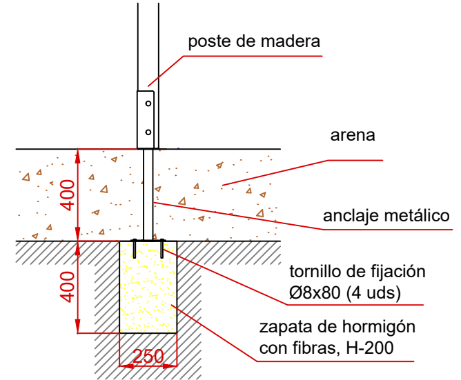
ESQUEMA DE CIMENTACIÓN EN ARENA E: 2/1
