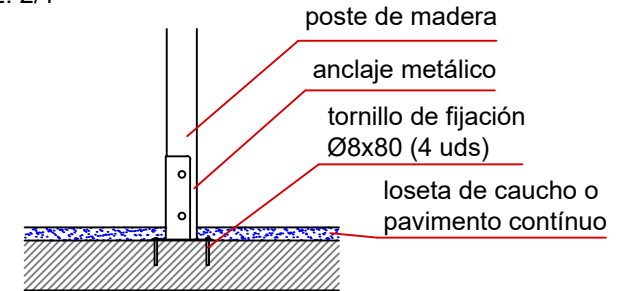
ESQUEMA DE CIMENTACIÓN EN HORMIGÓN E: 2/1
