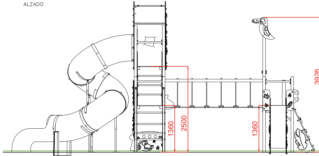
ALZADO
