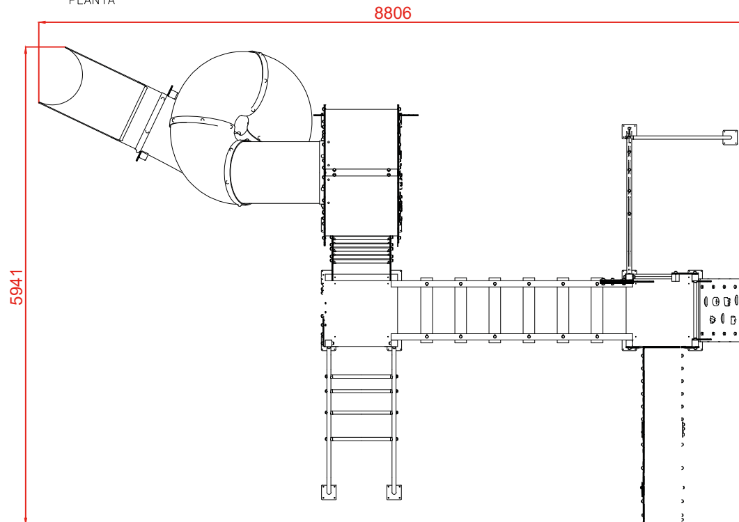
PLANTA
