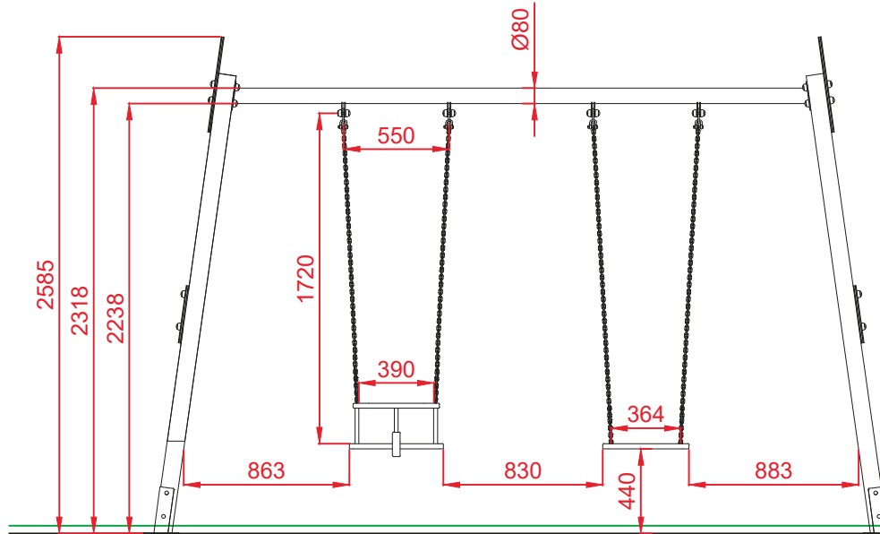
ALZADO
