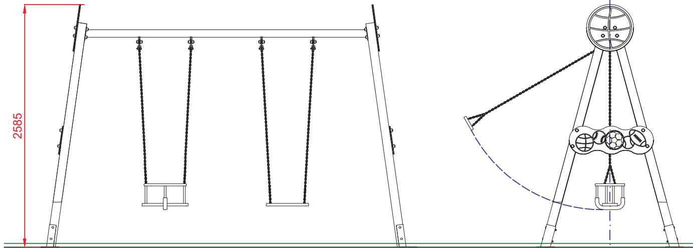
ALZADO
