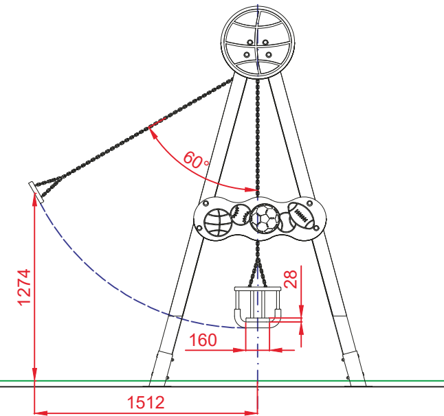
PERFIL IZQUIERDO
