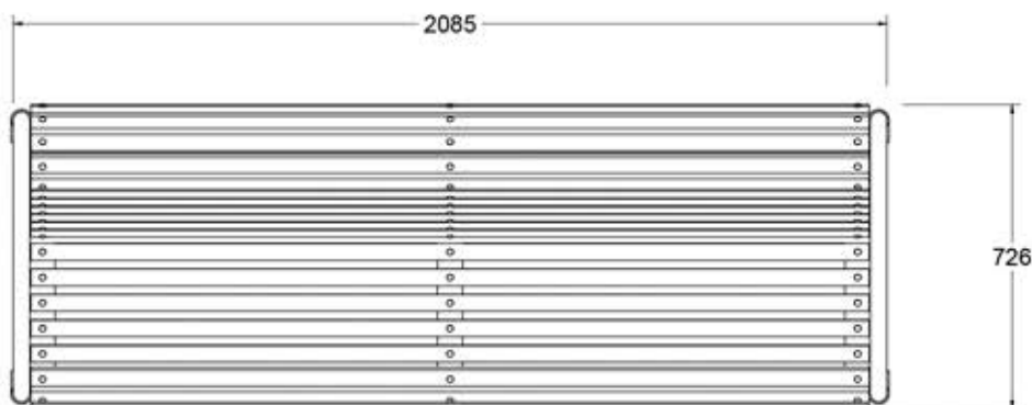
vista en planta 1:20
