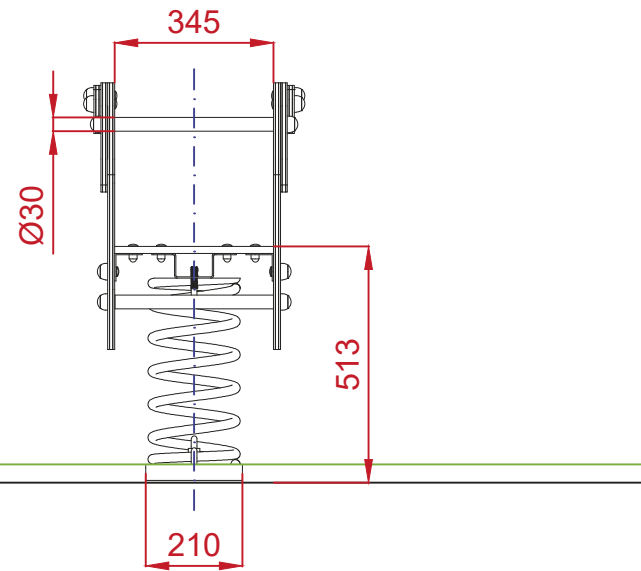
PERFIL
