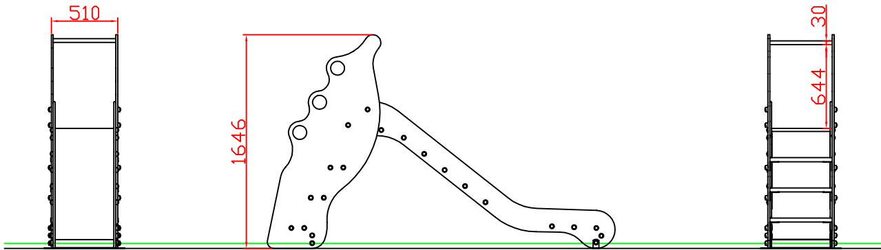
Perfil Izquierdo
