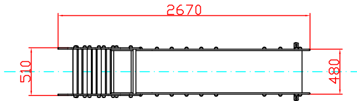
Alzado
