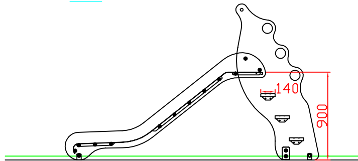
Planta
