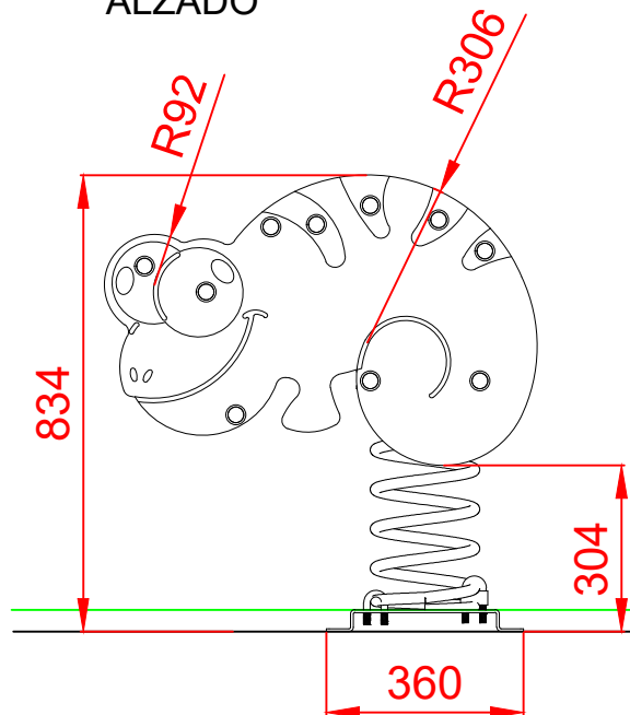
ALZADO
