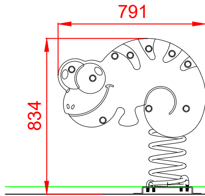
ALZADO
