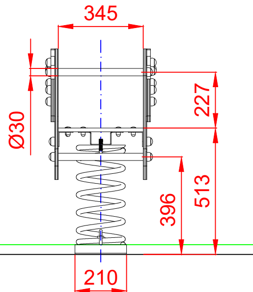
PERFIL
