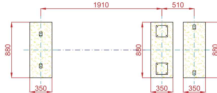
PLANTA CIMENTACIÓN
