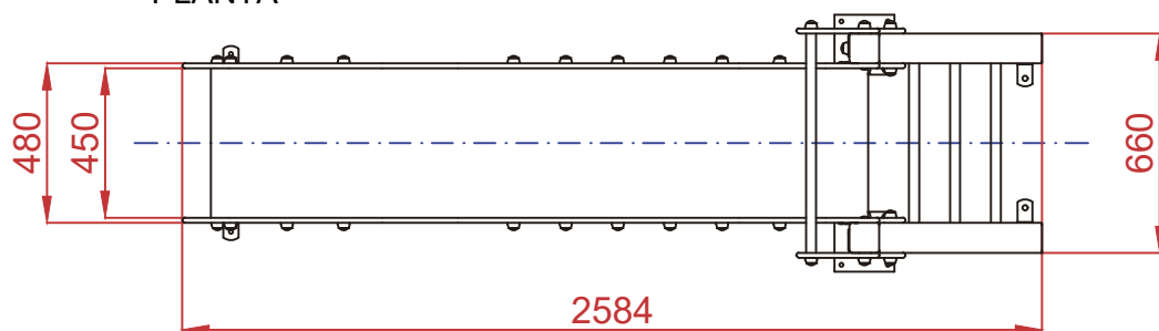
PLANTA
