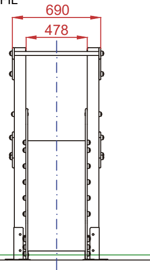
PERFIL
