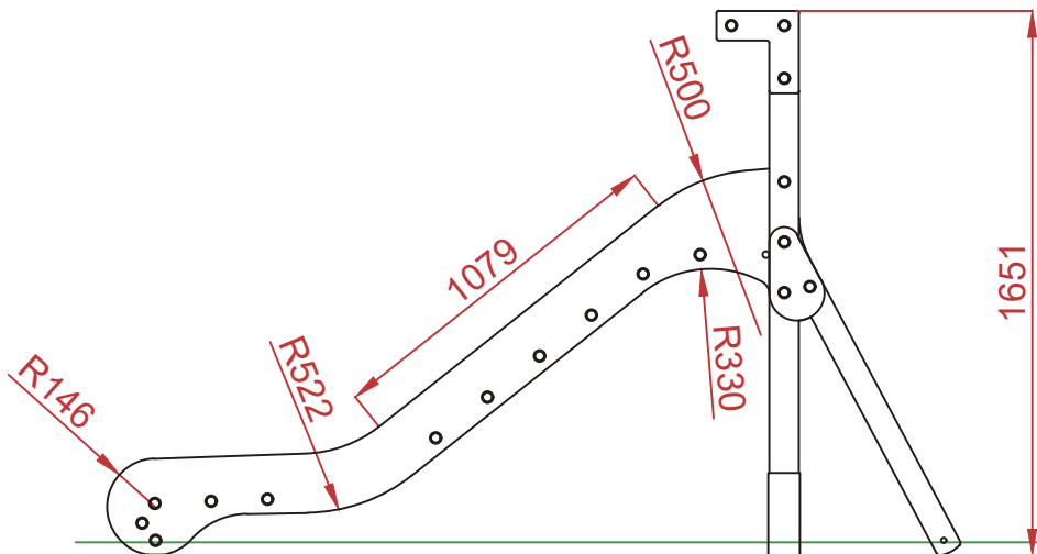
ALZADO
