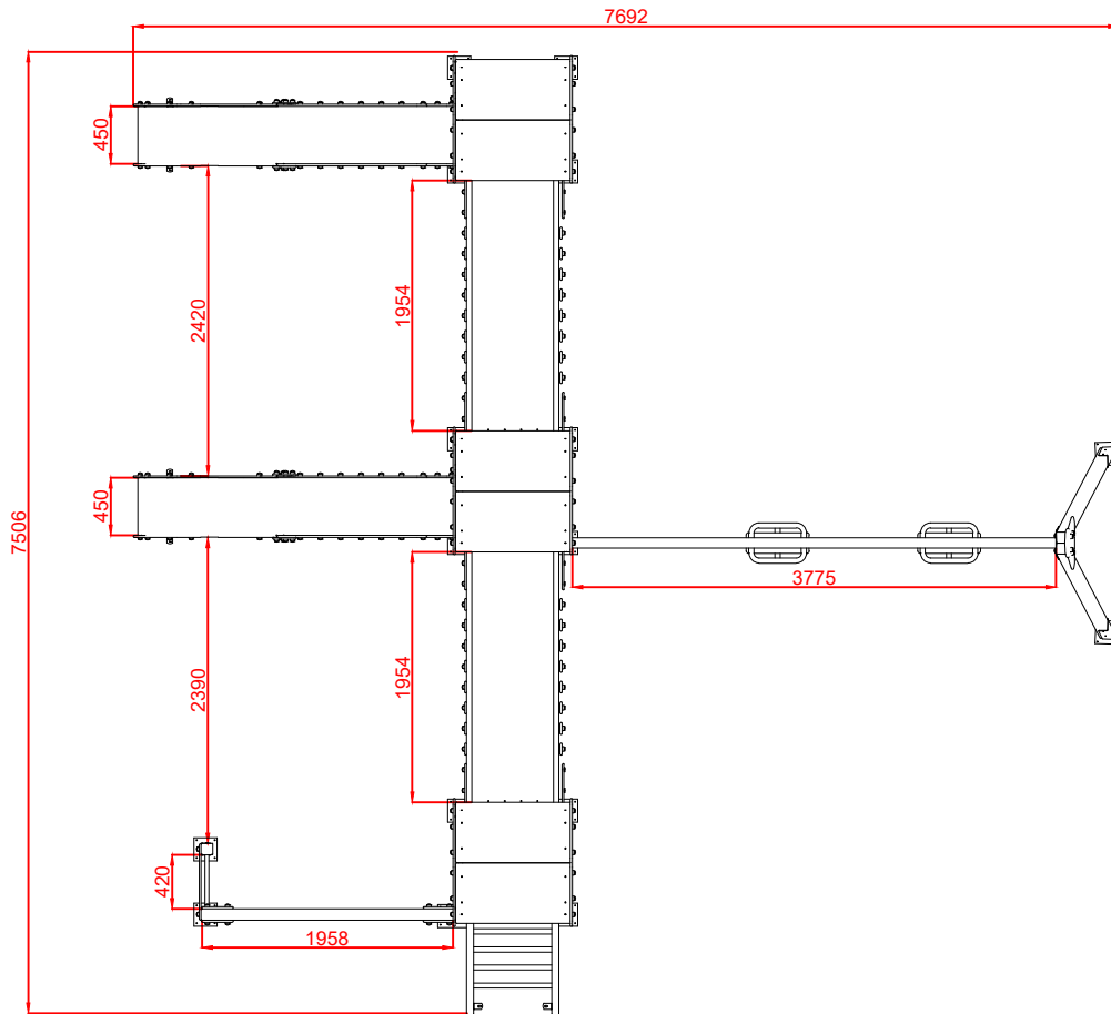
PLANTA
