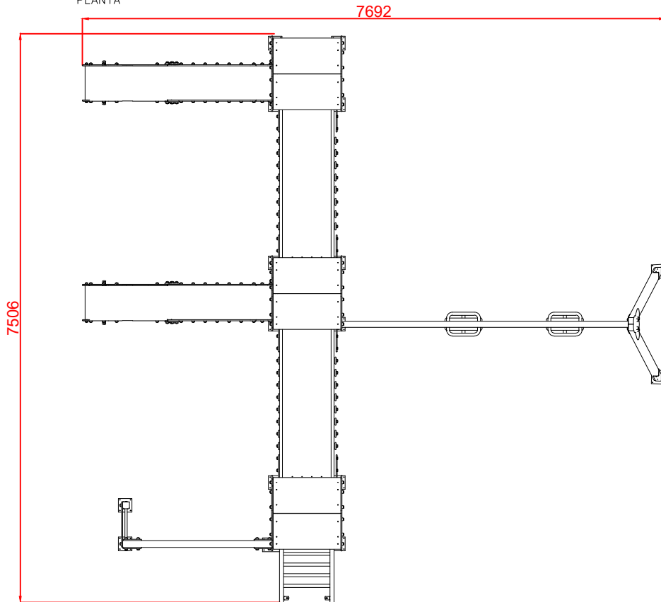
PLANTA
