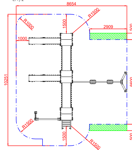
ÁREA DE SEGURIDAD ÁREA= 75,31 m 2 E: 1/2
