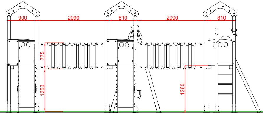
PERFIL IZQUIERDO
