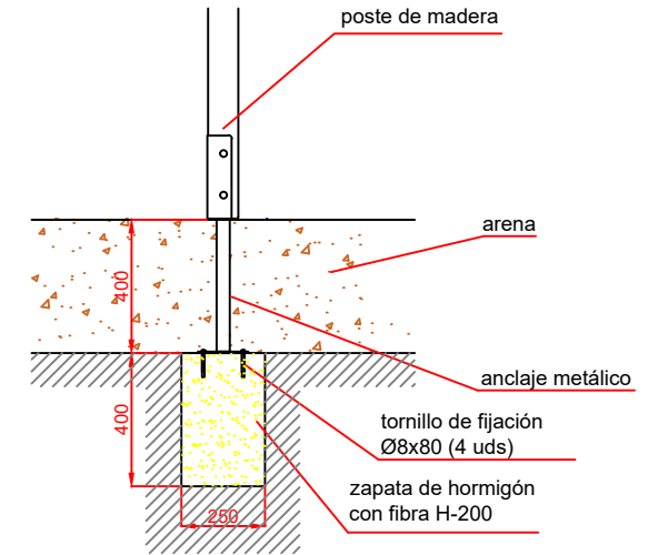
ESQUEMA DE CIMENTACIÓN EN ARENA E: 2/1
