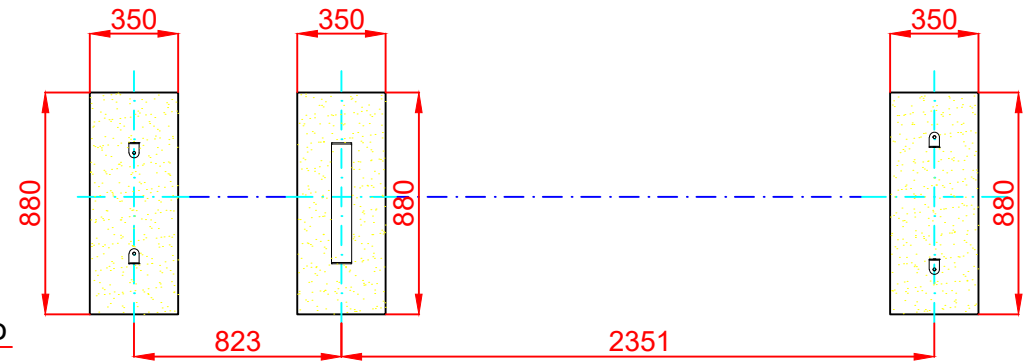
PLANTA CIMENTACIÓN
