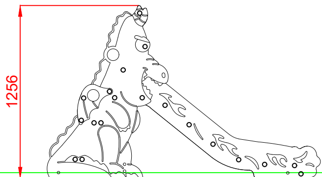
ALZADO
