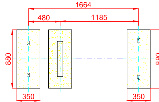
PLANTA CIMENTACIÓN
