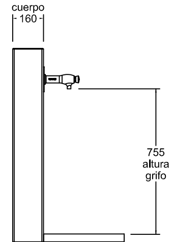
vista lateral 1:20
