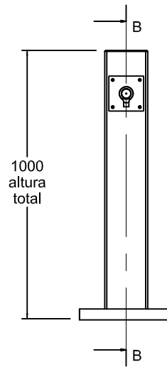
vista alzado 1:20
