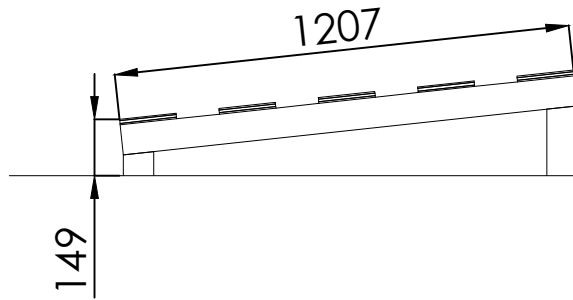
ALZADO
