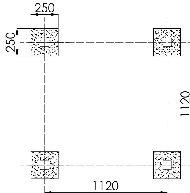
CIMENTACIÓN
