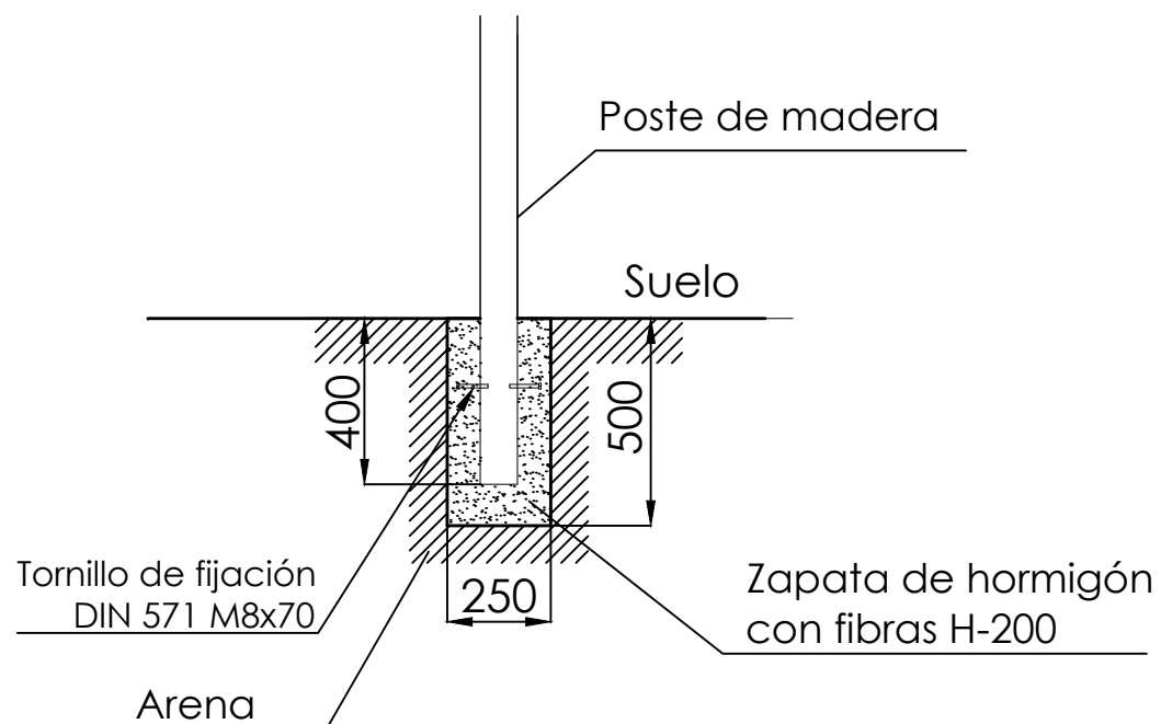
ESQUEMA DE CIMENTACIÓN
