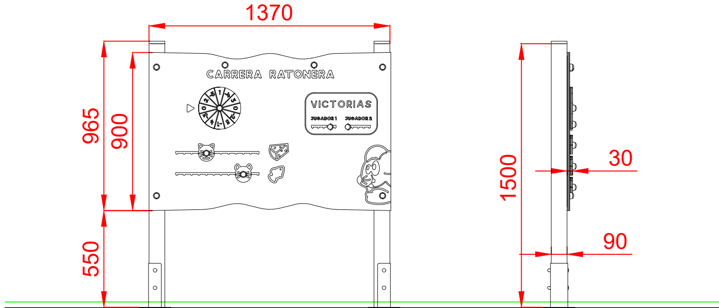
PERFIL IZQUIERDO
