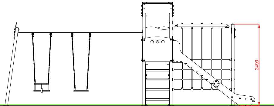
PERFIL IZQUIERDO
