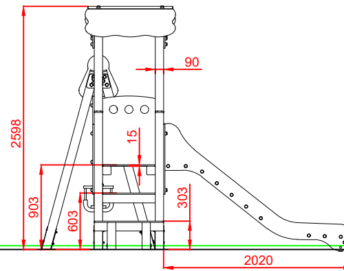
PERFIL IZQUIERDO
