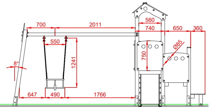
ALZADO POSTERIOR
